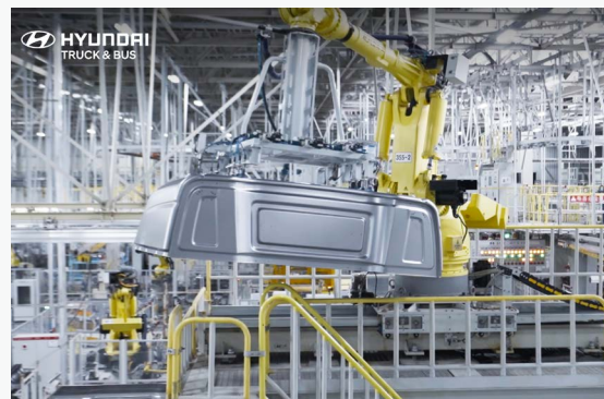
现代商用车智造工厂
